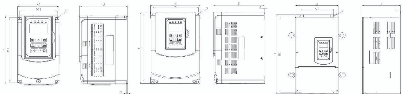
外型图 A
